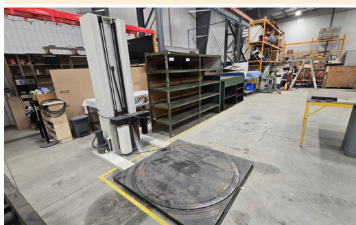
EMBALLEUSE À PALETTE MULLER, MOD. 301, SÉRIE 85401190, 120 V AVEC PLATEAU ROTATIF HAUTEUR AJUSTABLE
