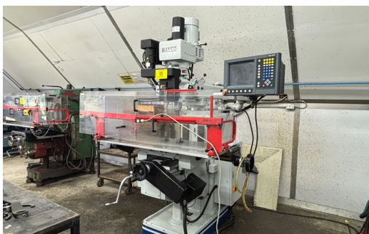
FRAISEUSE MILLING À TOURELLE DAVCO, 3 AXES, CONTRÔLE ACU-RITE
