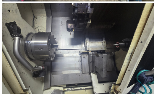
TOUR CNC DMG MORI SEIKI, CTX 510 ECONOLINE, CONTRÔLE SLIM LINE, 2013, OPTION AXE Y ET LIVE TOOLS, OUTILLAGE CÔNES 40
